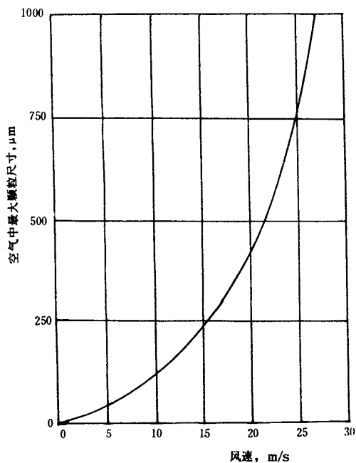
图 2 最大颗粒尺寸与风速的依赖关系 注:对最大粒子尺寸有影响的近地面条件(小于 1 m)的曲线
