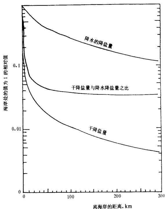
图 C1 推算干降盐量与降水降盐量及两者之比随离海岸远近的变化
